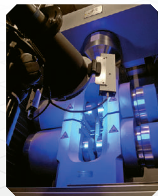
Extensomètre vidéo
