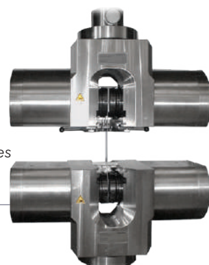
Outillages pour les essais de pliage
