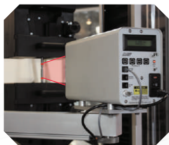
Extensomètre laser
